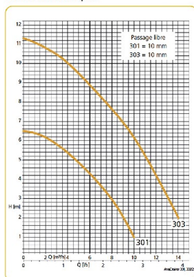
Courbes caractéristiques
